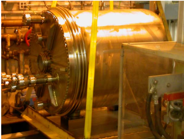
15-T solenoid in test location at MIT
