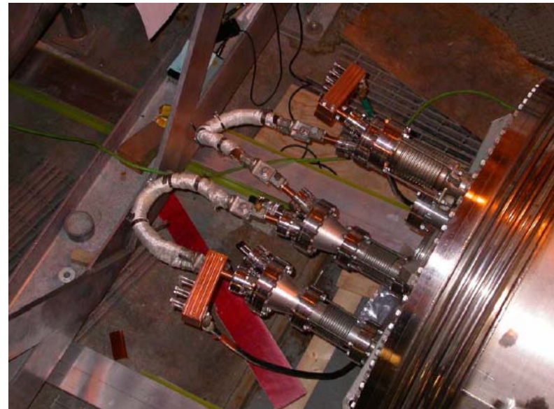
15-T solenoid in test location at MIT
